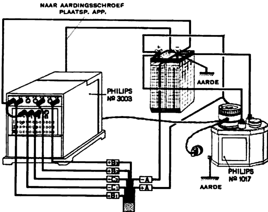
Fig. 3 Bij gebruik van Philips plaatspanningapparaat No. 3003 en Philips gelijkrichter No. 1017 (De neg. roosterspanning van bus -I is op -4 V, van bus -II op -15 V ingesteld)
