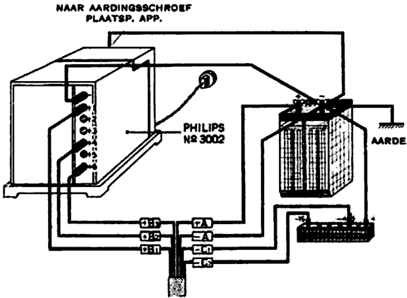
Fig. 5 Bij gebruik van Philips plaatsspanningapparaat No. 3002 met een batterij voor negatieve roosterspanning
