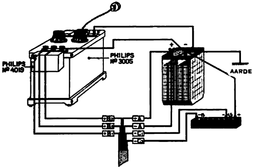
Fig. 7 Bij gebruik van Philips plaatsspanningapparaat No. 3005 („VOLT“-knop op stand „7“, „DET“-knop op stand III) met voorzetapparaat No. 4019 en met een batterij voor negatieve roosterspanning.
