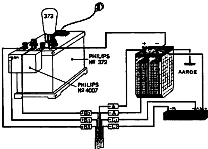
Fig. 6 Bij gebruik van Philips plaatsspanningapparaat No. 372 („VOLT“-knop op stand „MAX“, „DET“-knop op stand III) met voorzetapparaat No. 4007 en met een batterij voor negatieve roosterspanning
