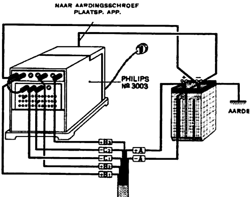
Fig. 4 Bij gebruik van Philips plaatspanningapparaat No. 3005 (De neg. roosterspanning van bus -I is op -4 V, van bus -II op -15 V ingesteld)
